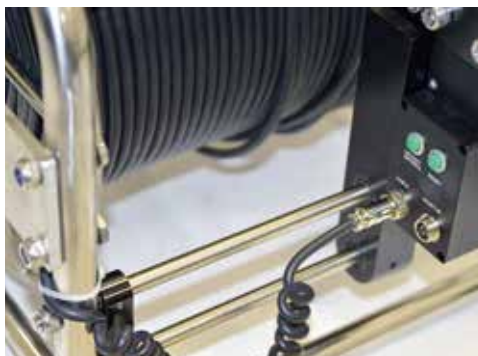
配管用工業内視鏡カメラシステム 120 メートル 型番 : PIP120HK
